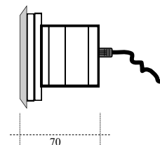
BOITIER D'ENCASTREMENT PROJECTEUR 6*3W
